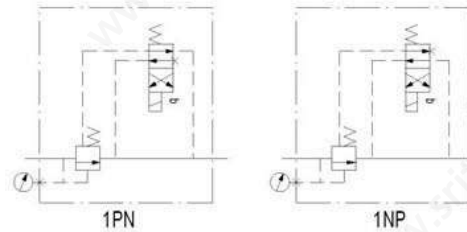
閥類型符號 SYMBOL SBSG-※
